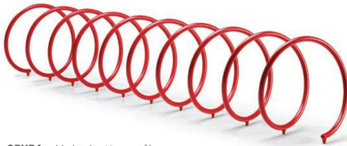
SPYRA sykkelstaiv. 40mm stålrør. Sandblåst, sinkprimet og pulverlakkert. 238 x 78 x 75cm
